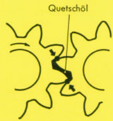
Bild 3 Quetschöl in den Zahnücken einer Zahnradpumpe (die kurzen Pfeile zeigen auf die abdichtenden Stellen)
