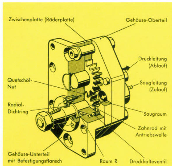
Bild 2 Bosch-Plattenpumpe HY/ZE ..
